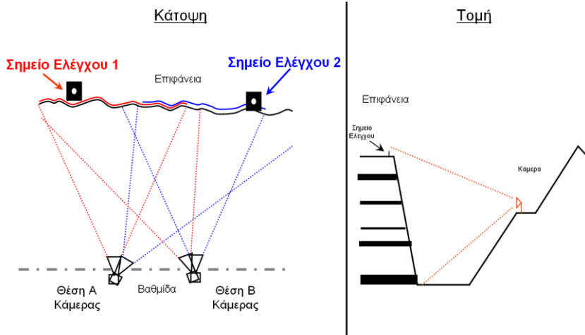
Σχήμα 2.5 Αρχή φωτογραμμετρίας
